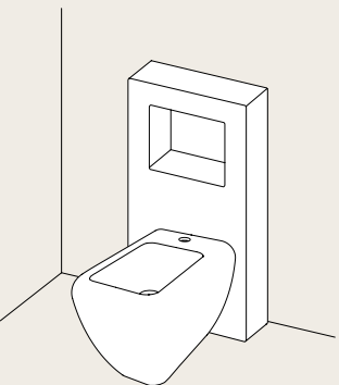
cassetta Magic-Box per vaso e bidet con vano portaoggetti Magic Cistern-box for wc pan and bidet with shelf 41,5 x 12 x 80h - MABX + SHVA-SHBI
