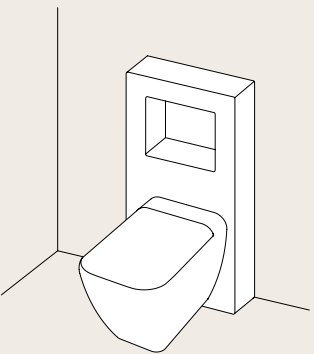
cassetta Magic-Box per vaso e bidet con vano portaoggetti Magic Cistern-box for wc pan and bidet with shelf 41,5 x 12 x 80h - MABX + SHVA-SHBI
