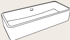
lavabo d'appoggio rettangolare 100 con troppopieno on top rectangular washbasin 100 with overflow 100 x 42 x h20 - SHLAA10020 pag. 152
