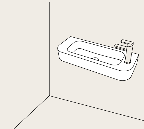
installazione sospesa con rubinetto da lavabo dx suspended installation with taps for washbasin dx 80 x 30 x h12 - SHSL80
