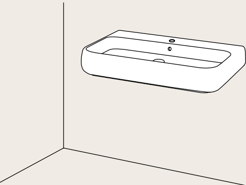
installazione sospesa wall-hung installation 80 x 48 x 15h - SHLS80
