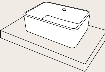
installazione da appoggio su piano on top installation 60 x 42 x h20 - SHLAA6020
