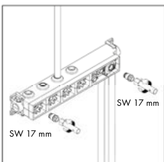
Remove the plug.
